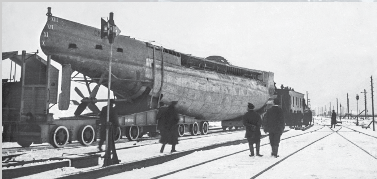
Подводная лодка «Скат» на железнодорожном транспортёре по пути на Дальний Восток. 1904 г. (ЦВММ)
