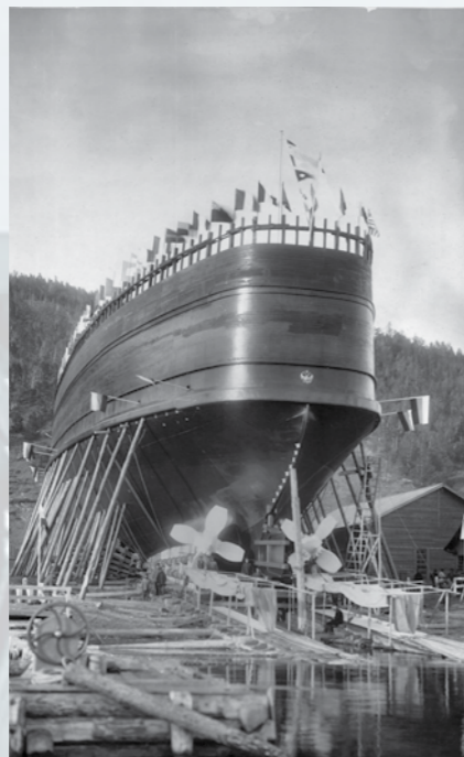
Ледокол «Байкал» на стапеле. «Альбом спуска паромо-ледокола Байкал 17 июня 1899 г. С. Лиственничное» (ЦМЖТ)
